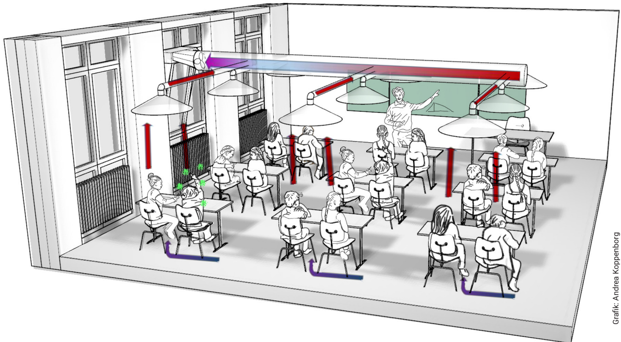
Schematische Darstellung der Abluftanlage in einem Klassenraum. | Schematic overview of the exhaust air system in a classroom.
